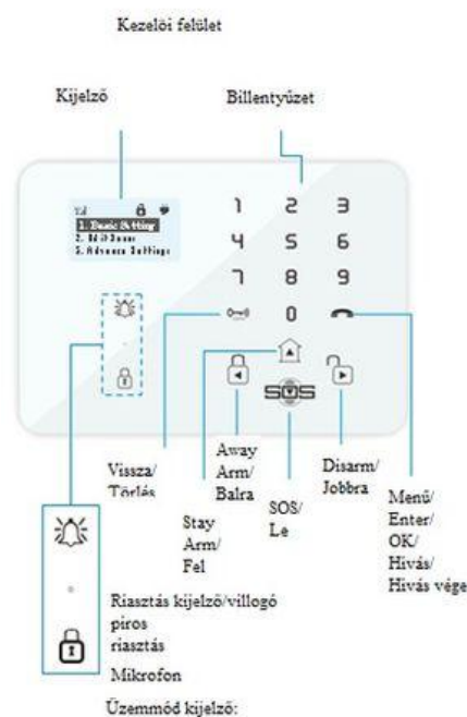
A főegység elől nézeti megjelenése
